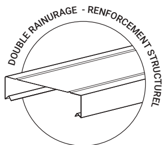
VUES TECHNIQUES COUVERTINE ALUMINIUM
